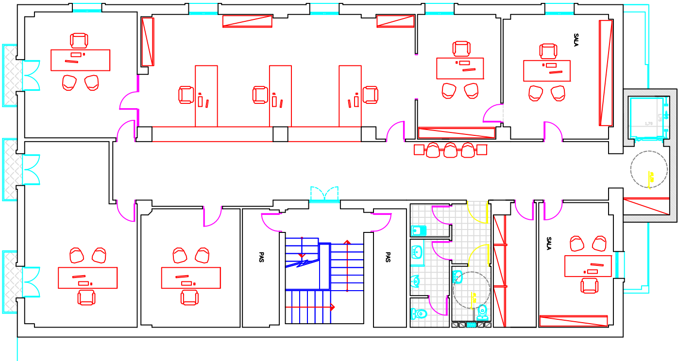
-PLANTA PRIMERA-
